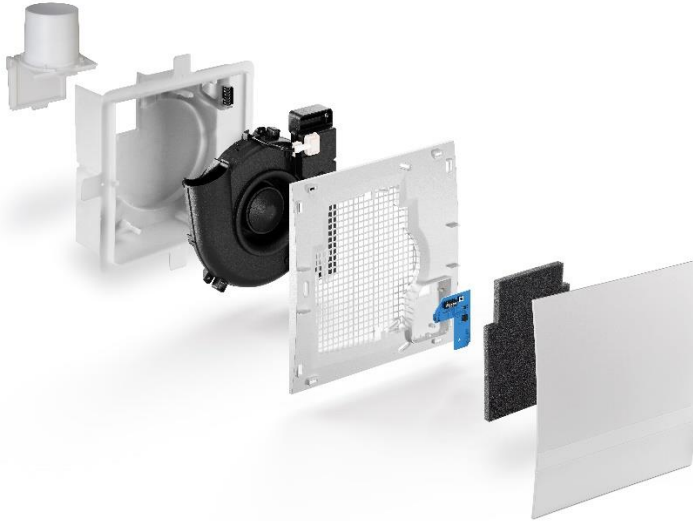
Abbildung: Der Silvento ec Typ V
