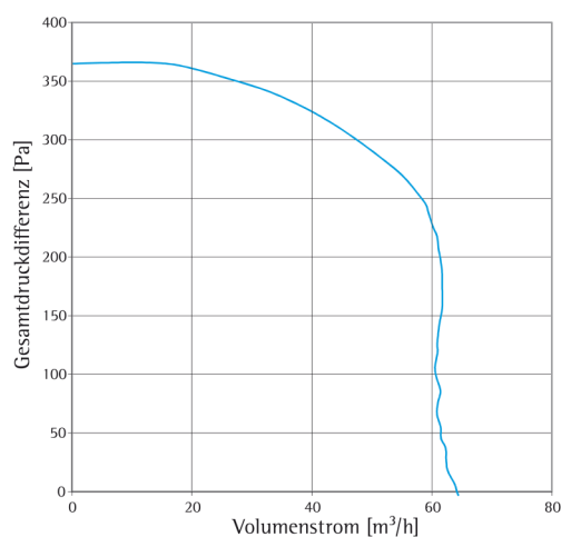
Druck-Volumen-Kennlinie UP-R
