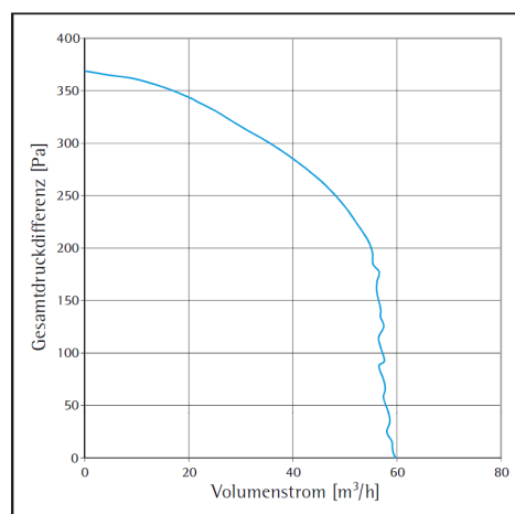
Druck-Volumen-Kennlinie 3/UP-2BR
