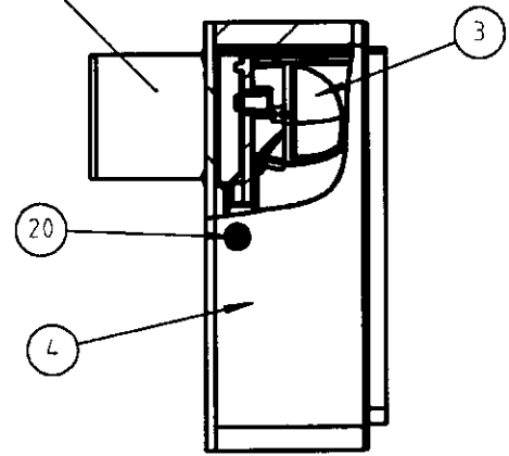
Brandschutz-Unterputzgehäuse 3/UP-BA
