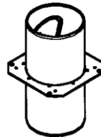
Absperrvorrichtung Silvento-BSK Typ 8/BS für Schachtwandmontage
