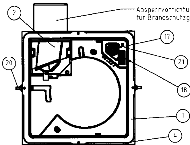
Brandschutz-Unterputzgehäuse 3/UP-BR
