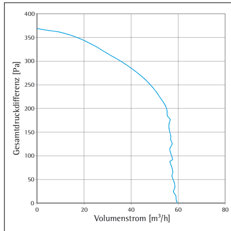
Druck-Volumen-Kennlinie UP-BR
