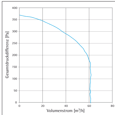
Druck-Volumen-Kennlinie AP
