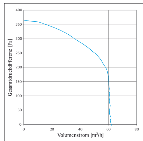
Druck-Volumen-Kennlinie AP-B
